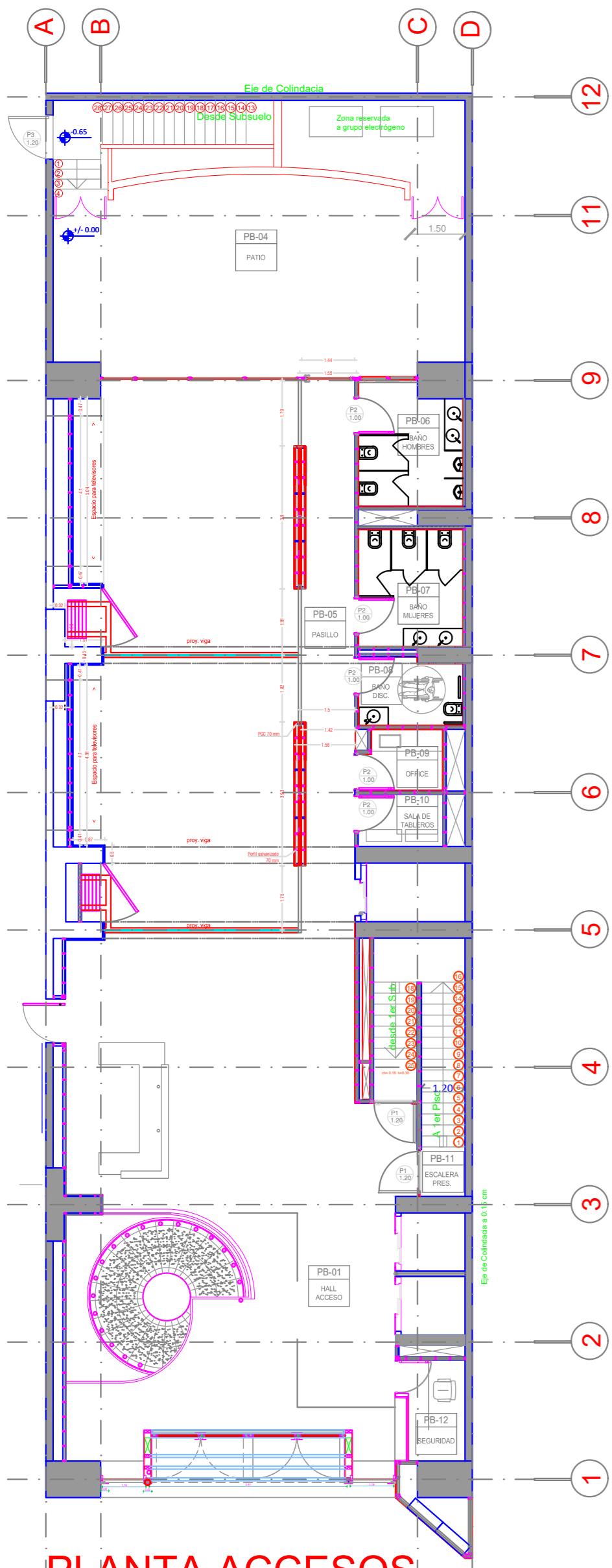
PLANTA ACCESOS SALAS REUNIONES
