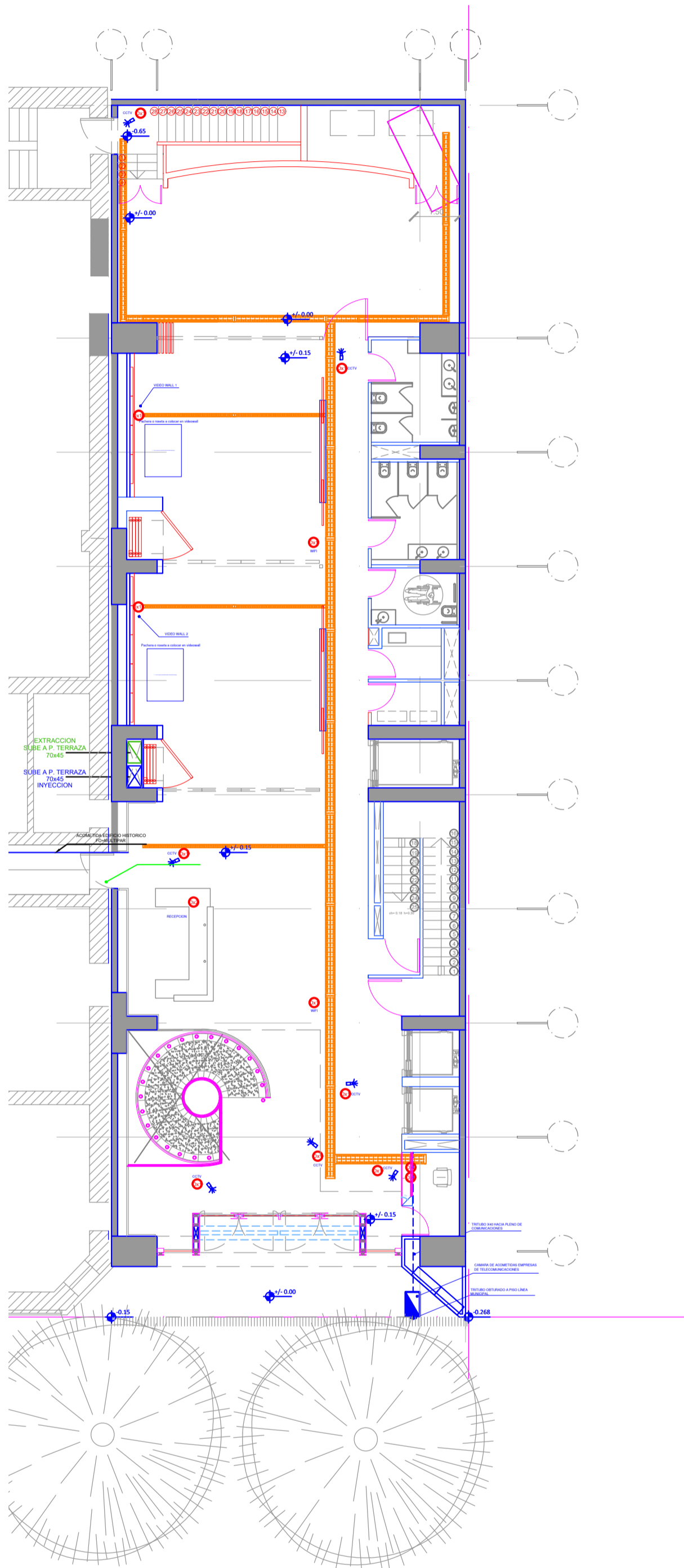
PLANTA ACCESOS SALAS REUNIONES
