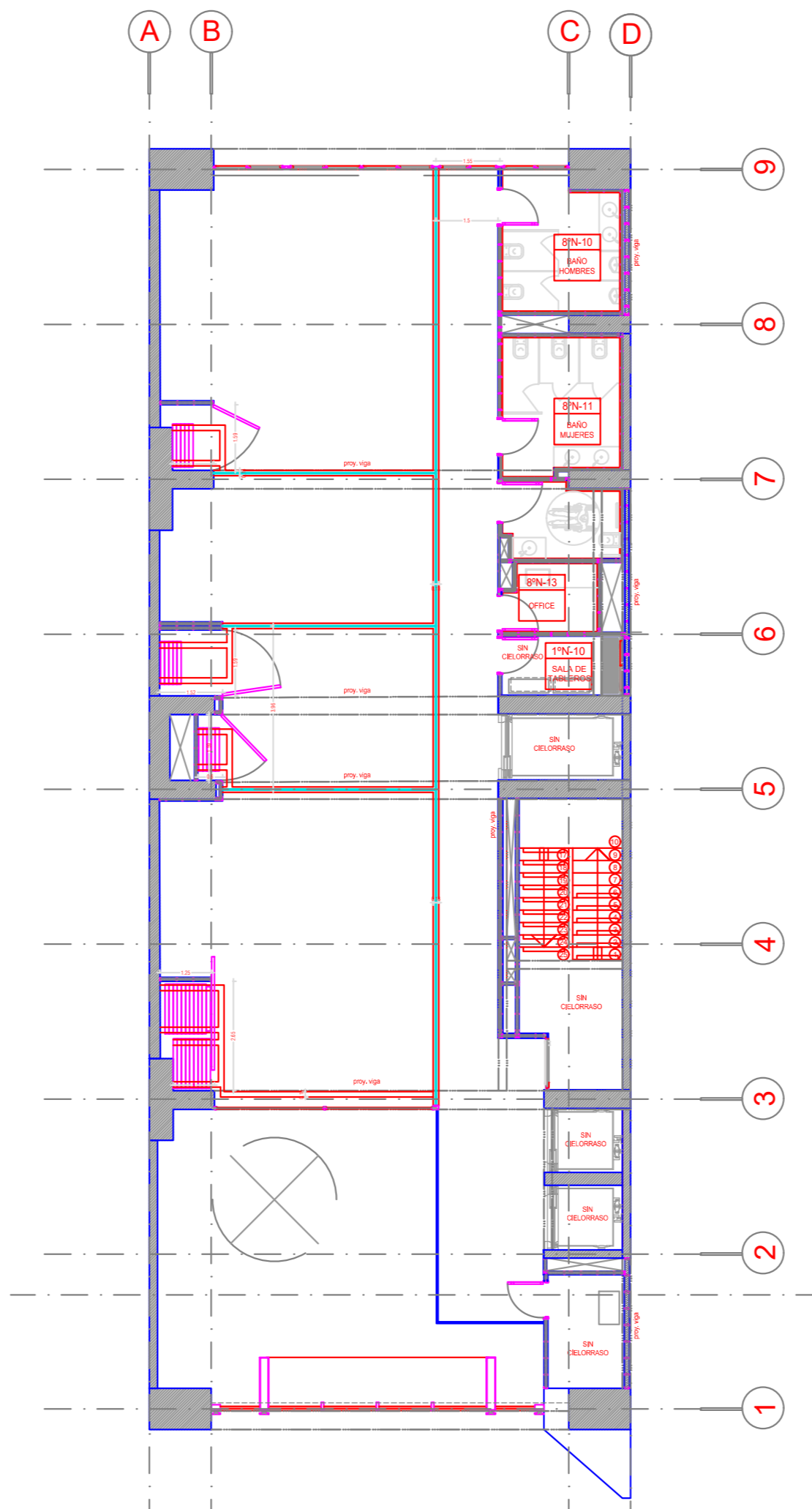
1° NIVEL (+ 4.50) BLOQUES
