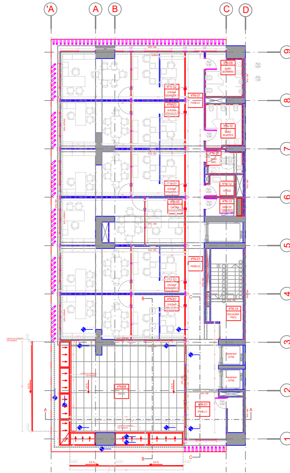
4° NIVEL (+ 15.00) OFICINAS SENADORES (6) PLAZA DE LOS SENADORES
