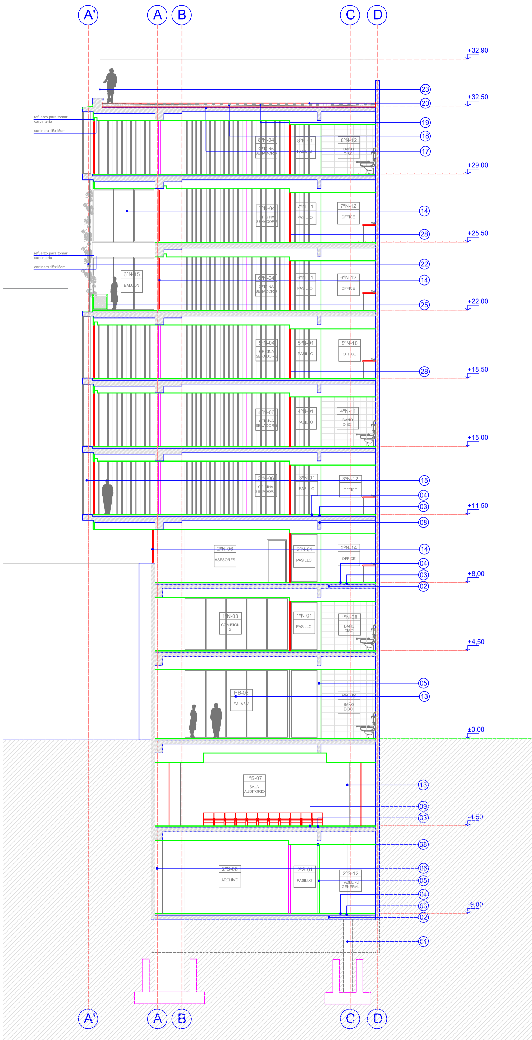
CORTE C-C
