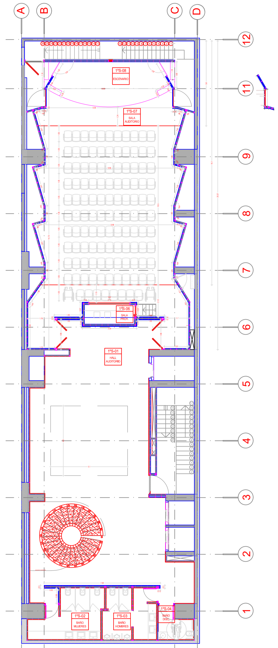
PLANTA 1ER SUBSUELO
