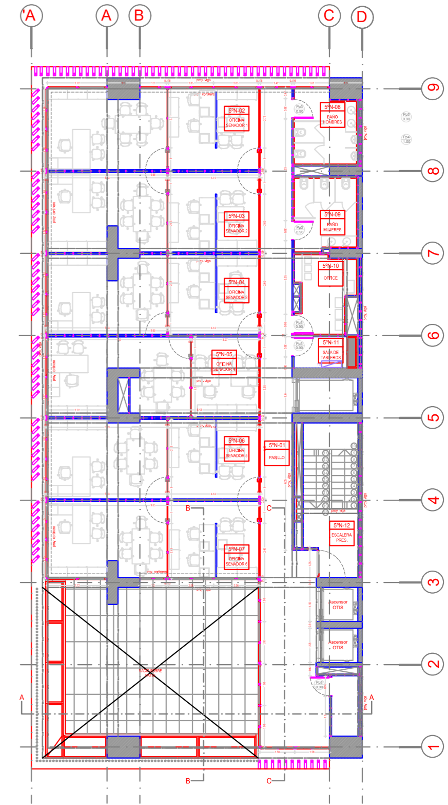
5° NIVEL (+ 18.50) OFICINAS SENADORES (6)
