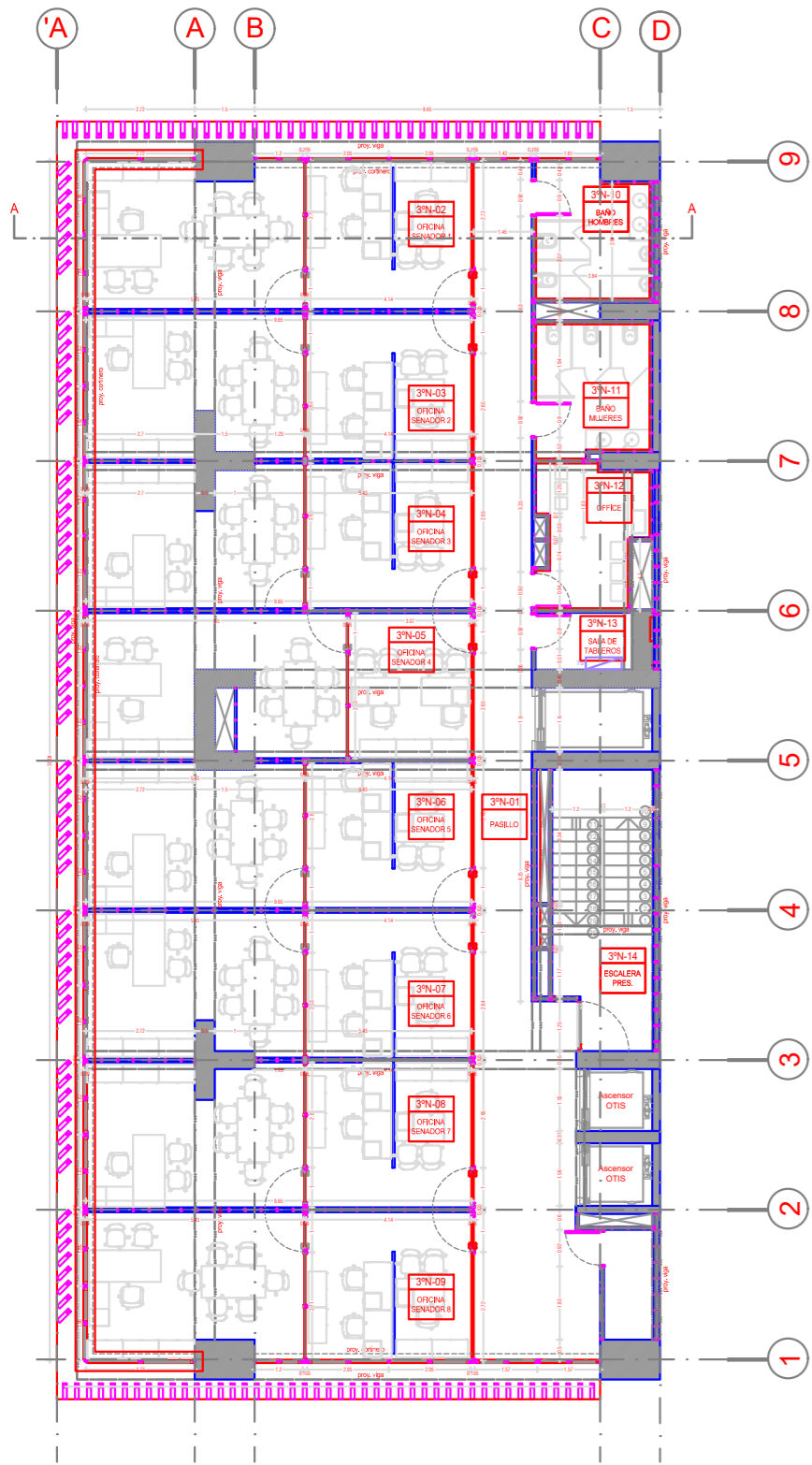
3° NIVEL (+ 11.50) OFICINAS SENADORES (8)
