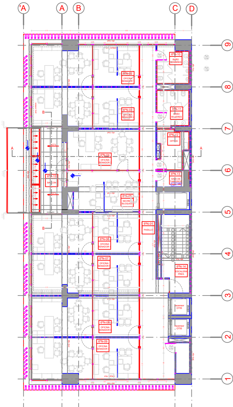
6° NIVEL (+ 22.00) OFICINAS SENADORES
