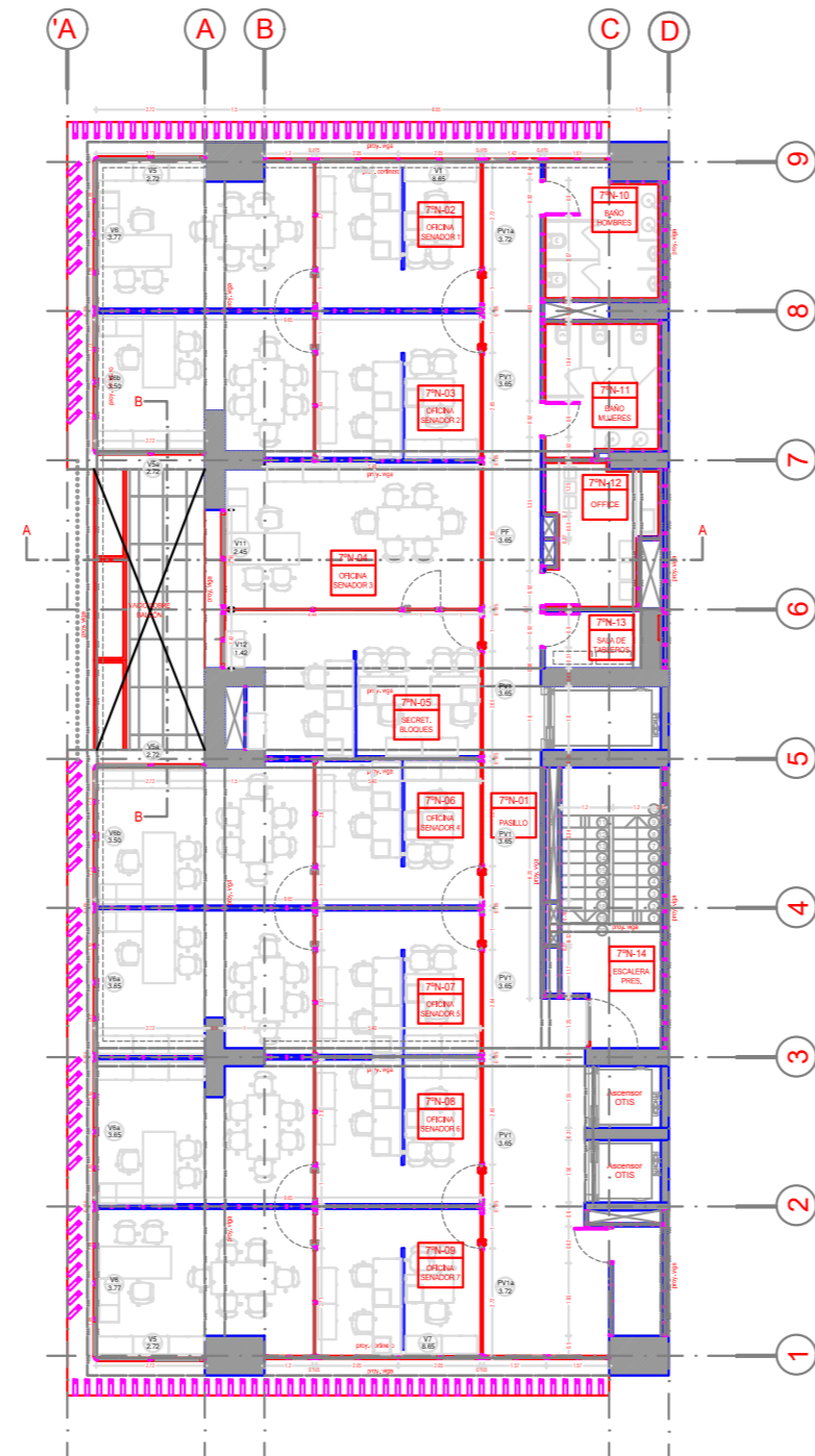
7° NIVEL (+ 25.50) OFICINAS SENADORES
